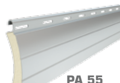
PA 55 inaltimea profilului: 55 mm grosimea: 14 mm
