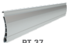
PT 37 inaltimea profilului: 37 mm grosimea: 8 mm
