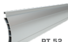
PT 52 inaltimea profilului: 52 mm grosimea: 14 mm
